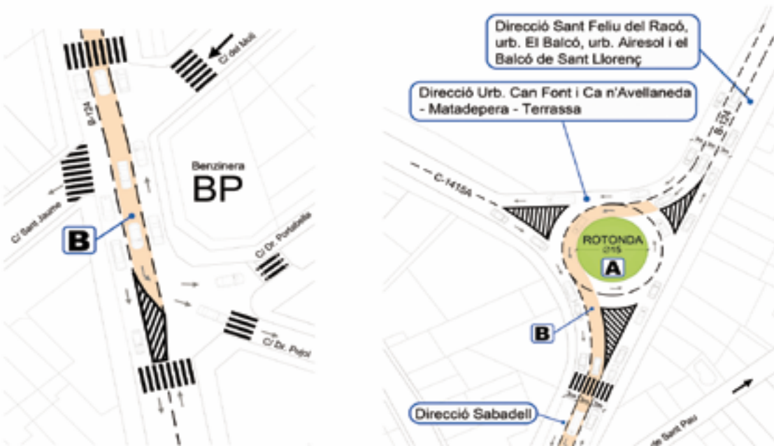
Al gràfic de l'esquerra (B) Tercer carril (Permet fer el gir cap els carrers Portabella i Pujol sense aturar els que van direcció a Sabadell) i al gràfic de la dreta, (A) Rotonda de 15m de diàmetre (la rotonda dona fluïdesa a la circulació en aquest punt) i B - Tercer carril. || CEDIDA
